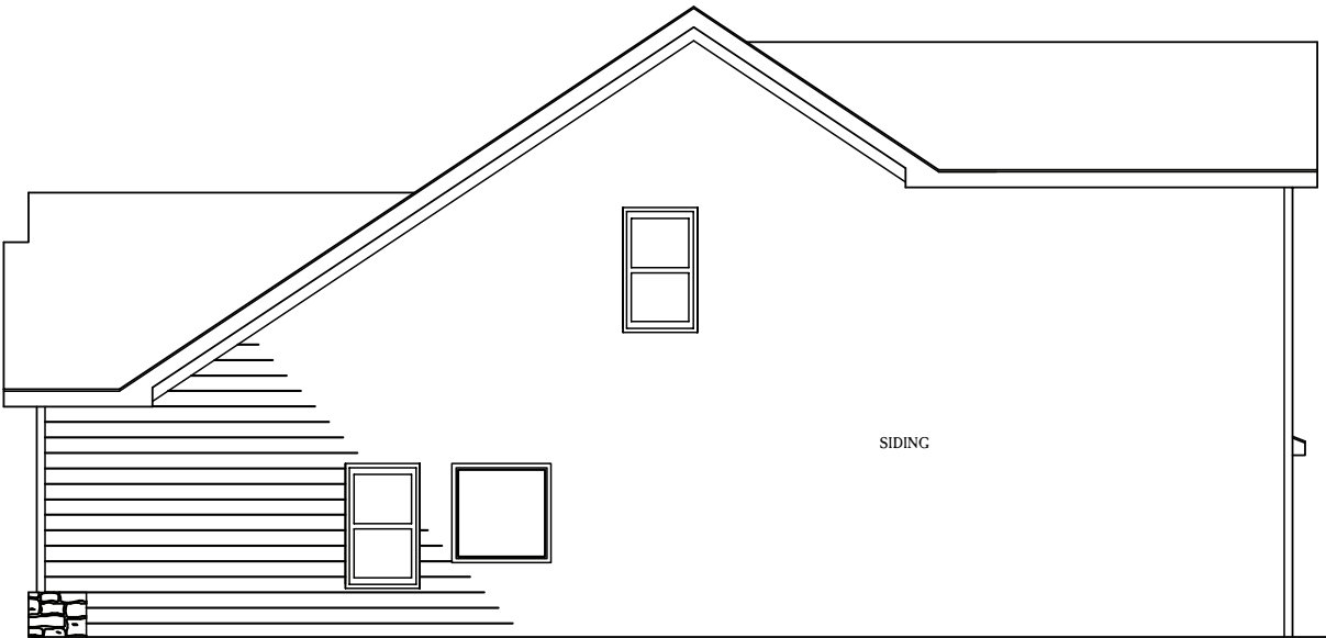
RIGHT ELEVATION
